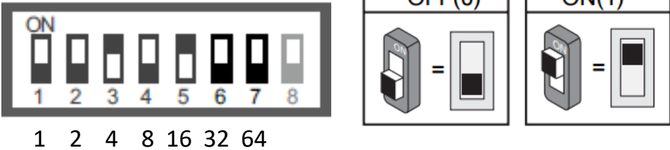
Switch d'adressage des postes
