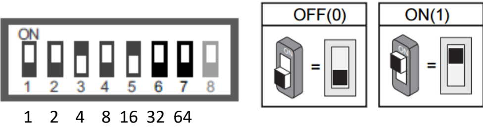
Switch d'adressage des postes
