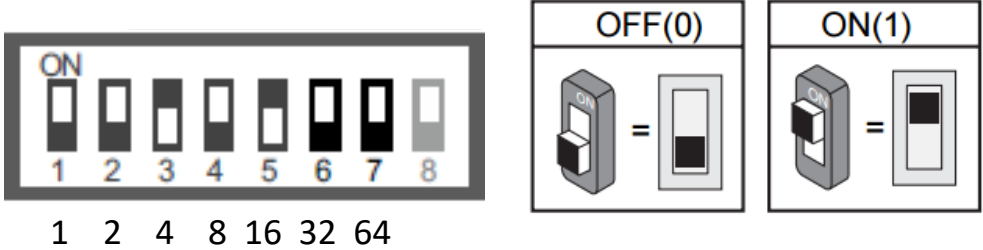
Switch d'adressage des postes
